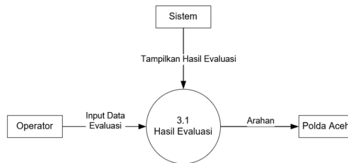
Gambar 6. DFD Level 3
