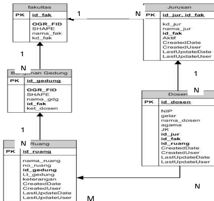
Gambar 2. Diagram Keterhubungan Anatartabel pada Sistem
